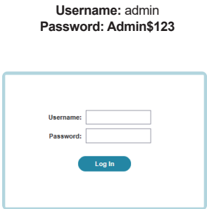
Figure 4. WebUI login
